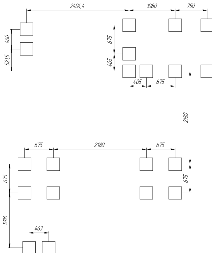
Рис.1. Схема бетонирования.
