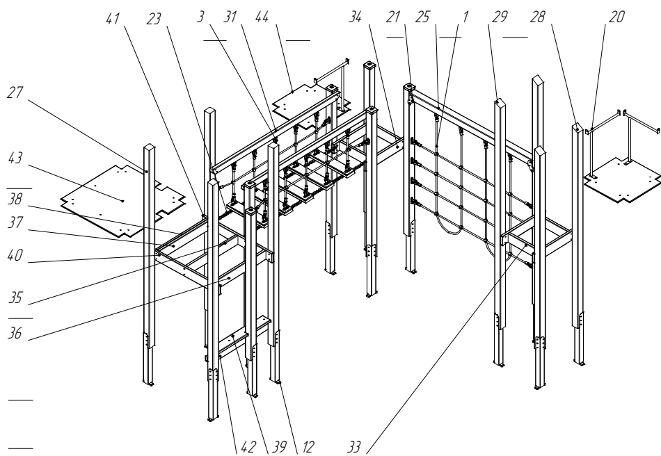
Рис 3.Схема сборки №1.
