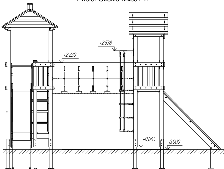
Рис.6. Схема высот 2.
