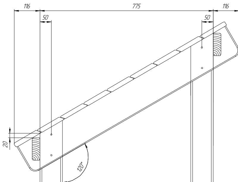
Рис.13. Схема установки односкатной крыши
