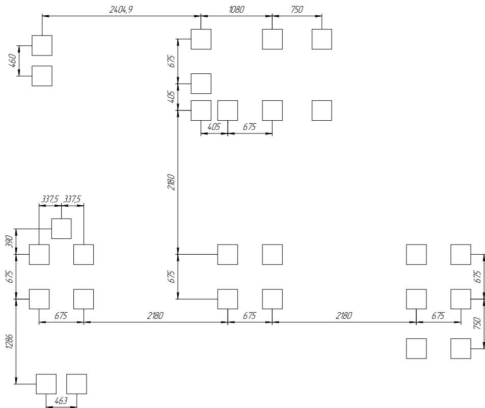
Рис.1. Схема бетонирования.
