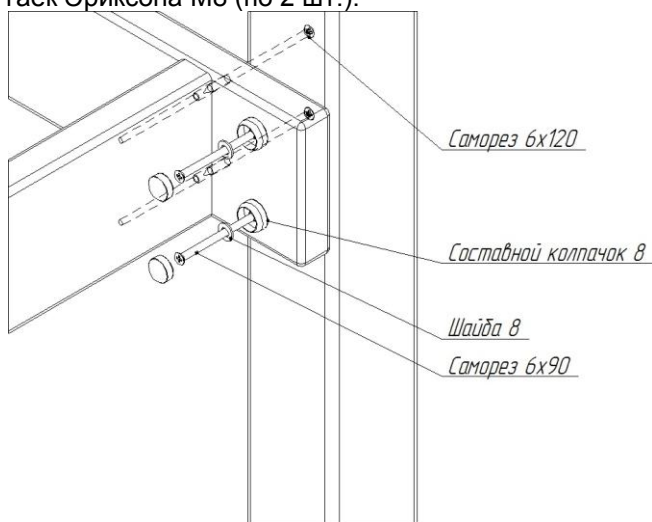
Рис.10. Схема сборки и установки каркаса.
