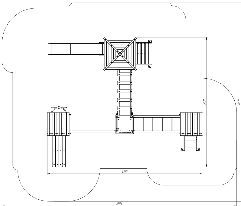
Рис.2. Схема зоны безопасности.
