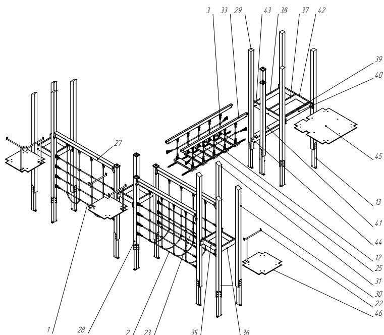
Рис 3.Схема сборки №1.
