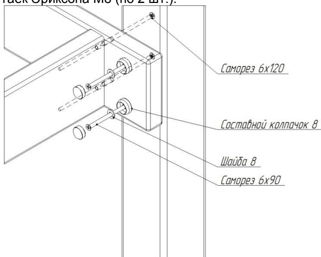
Рис.9. Схема сборки и установки каркаса.
