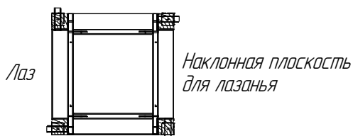
Рис.6. Схема расположения настила пола.
