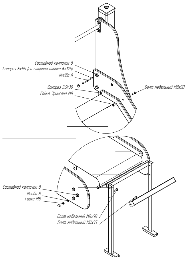
Рис.11. Схема сборки горки
