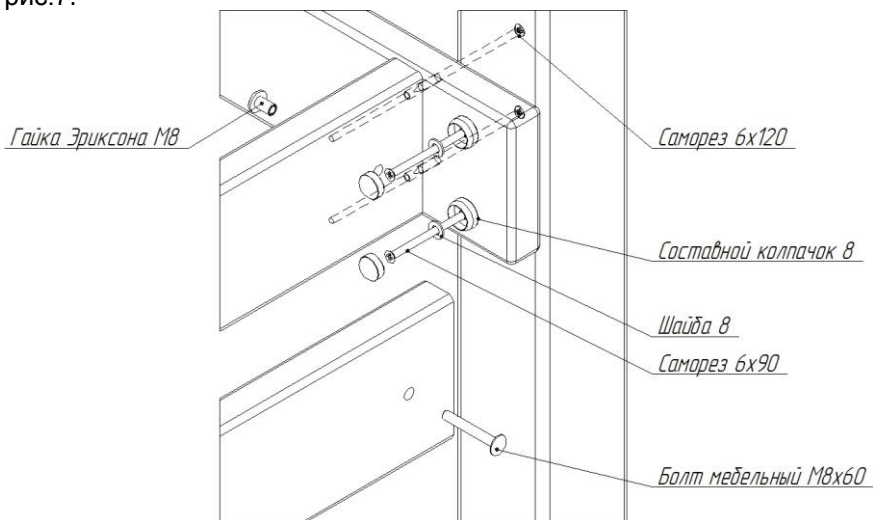
Рис.8. Схема сборки и установки каркаса с выходом на лестницу.
