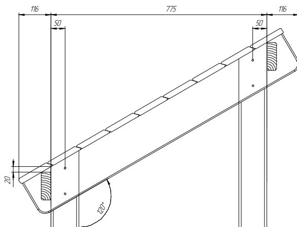
Рис.12. Схема установки односкатной крыши
