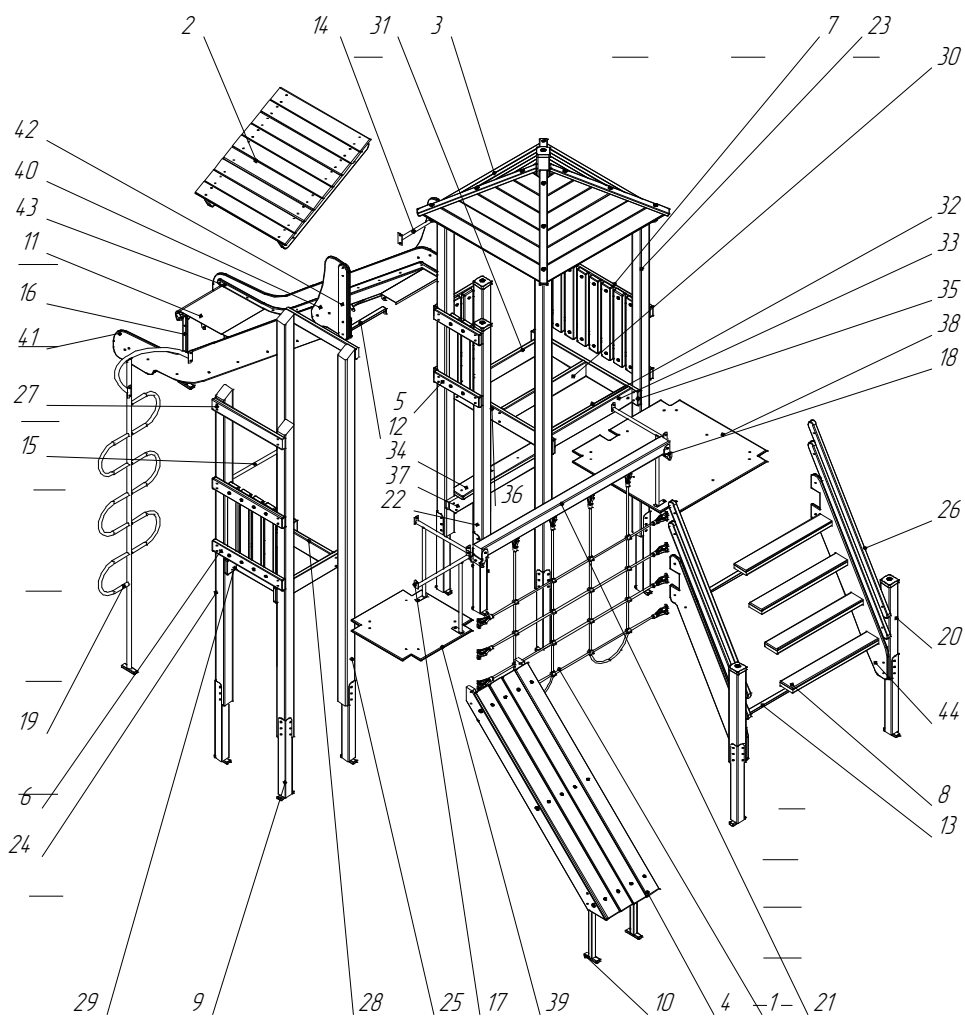
Рис 3.Схема сборки.
