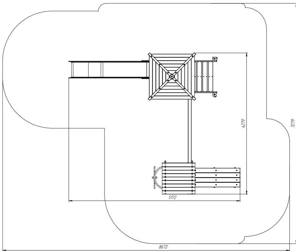
Рис.2. Схема зоны безопасности.
