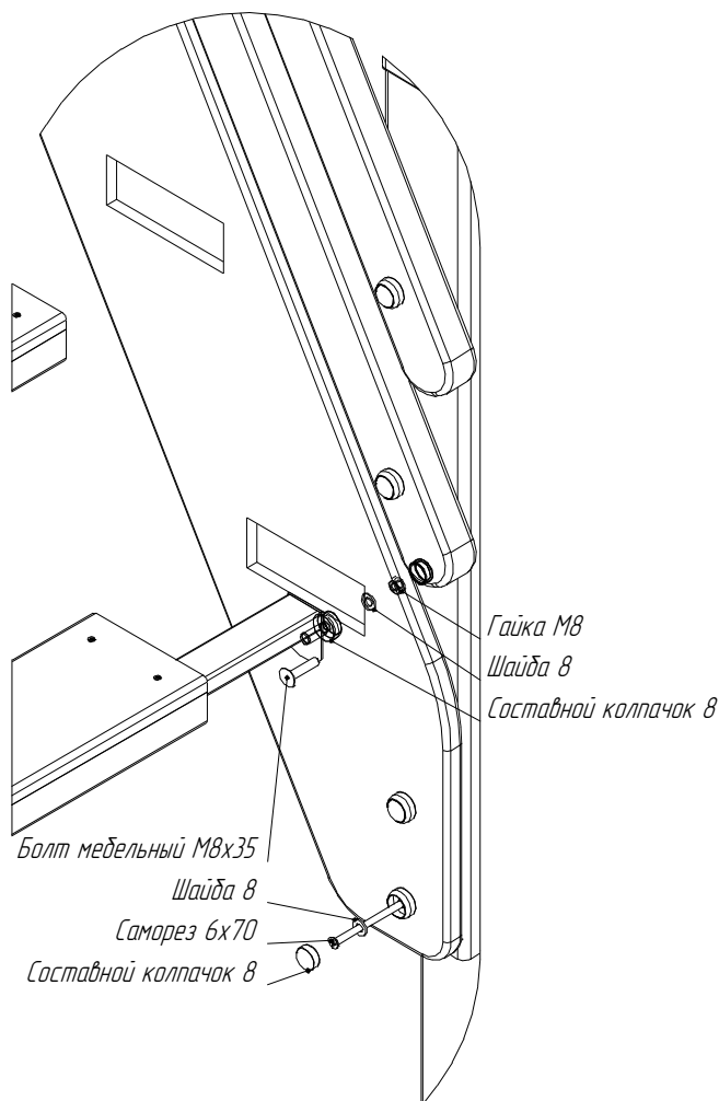
Рис.10. Схема сборки лестницы
