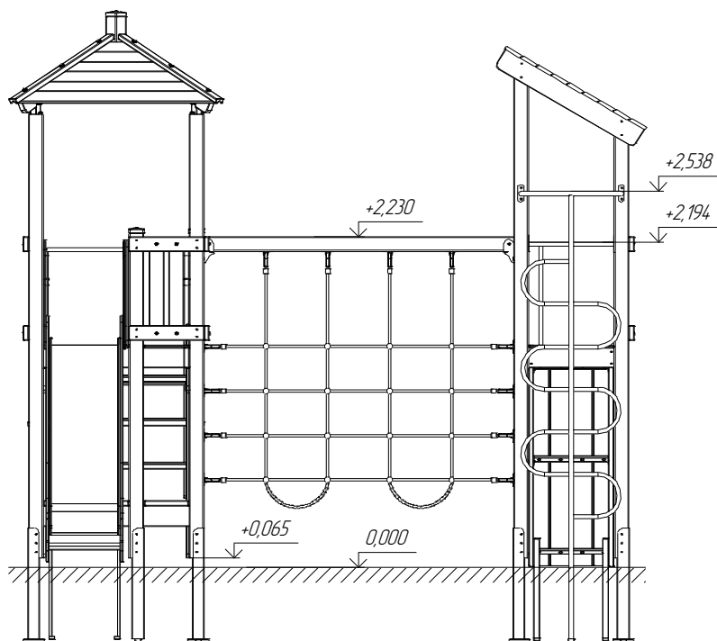
Рис.5. Схема высот 2.
