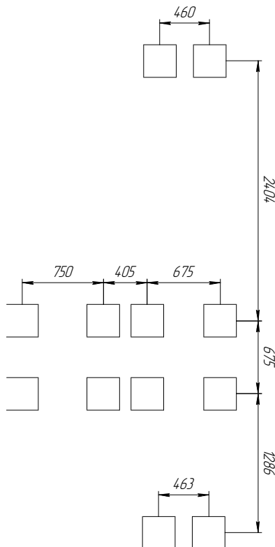
Рис.1. Схема бетонирования.
