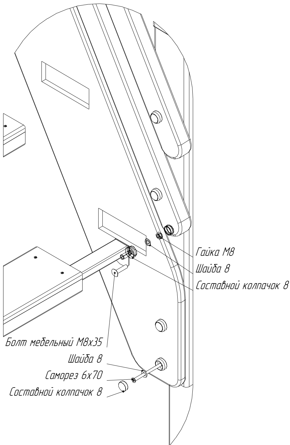
Рис.8. Схема сборки лестницы
