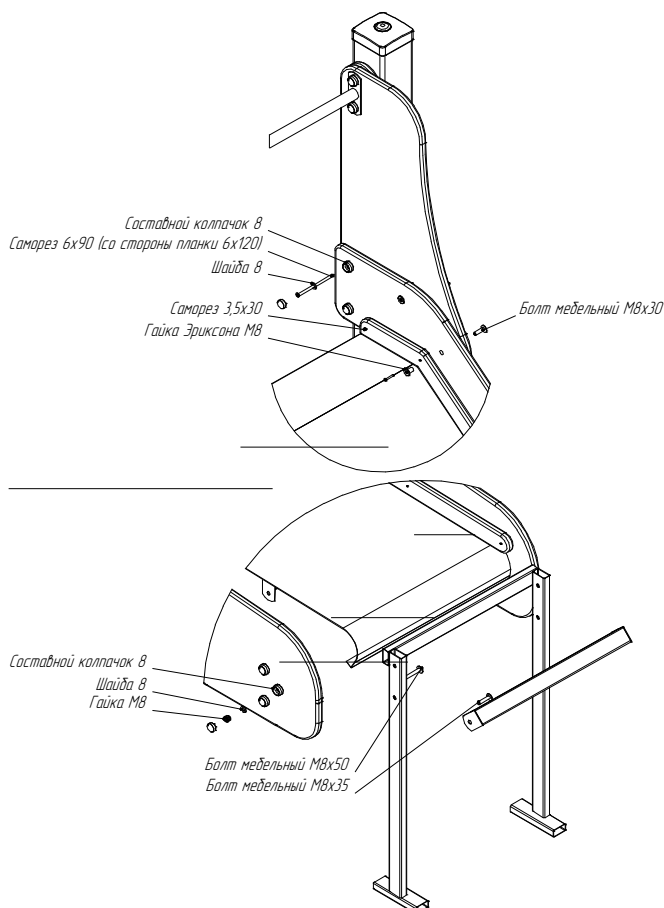
Рис.9. Схема сборки горки
