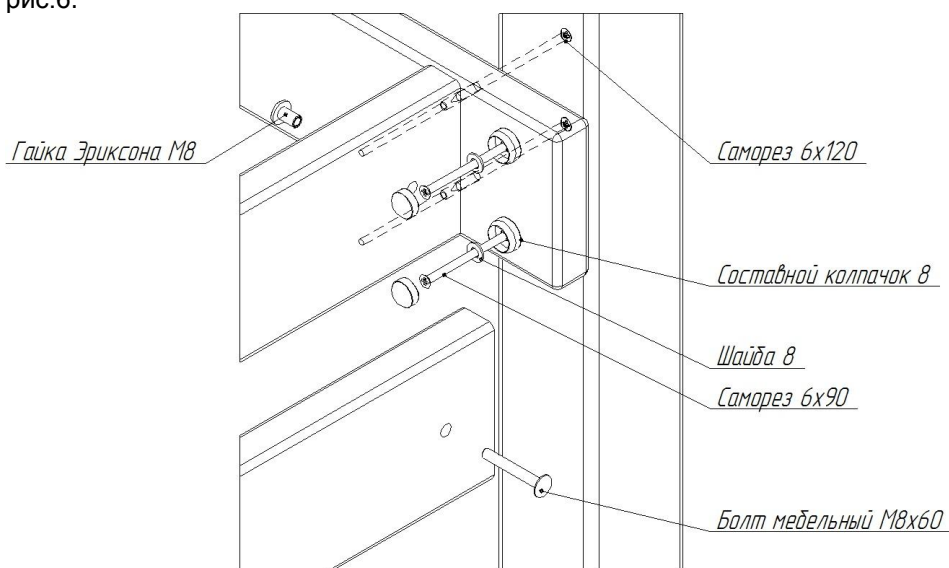
Рис.7. Схема сборки и установки каркаса с выходом на лестницу.
