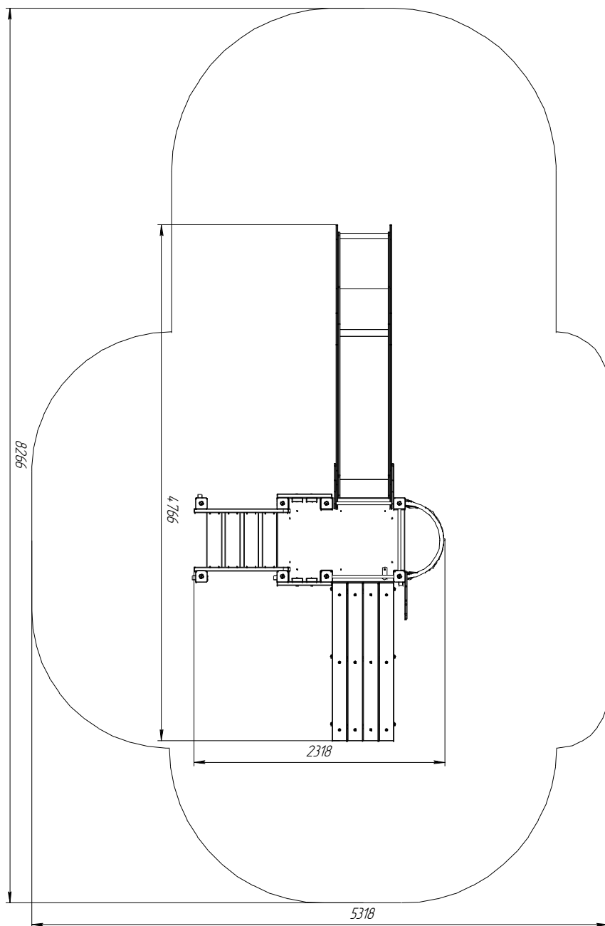
Рис.2. Схема зоны безопасности.
